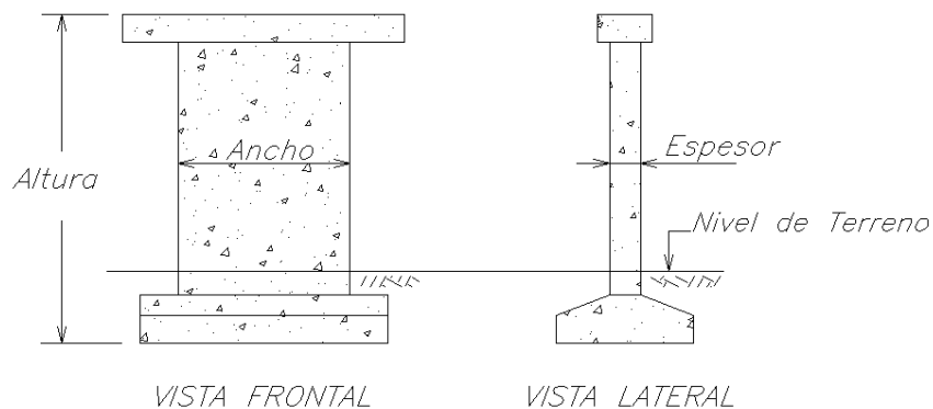
Figura 1.44 Pila tipo muro
