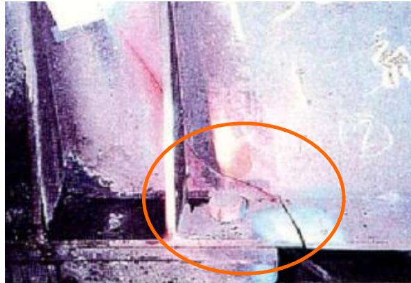
Figura 6-22 Grieta cerca del apoyo de la viga principal
