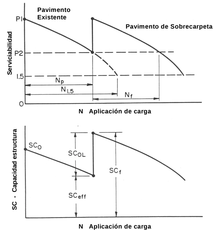
Figura 8-2 Pérdida de capacidad estructural después de tiempo y tránsito
