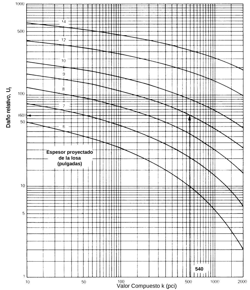
Figura 4-6 Cálculo del Daño relativo ( U_r ) en pavimento rígidos, en función del espesor de losa y Módulo de reacción de la subrasante
