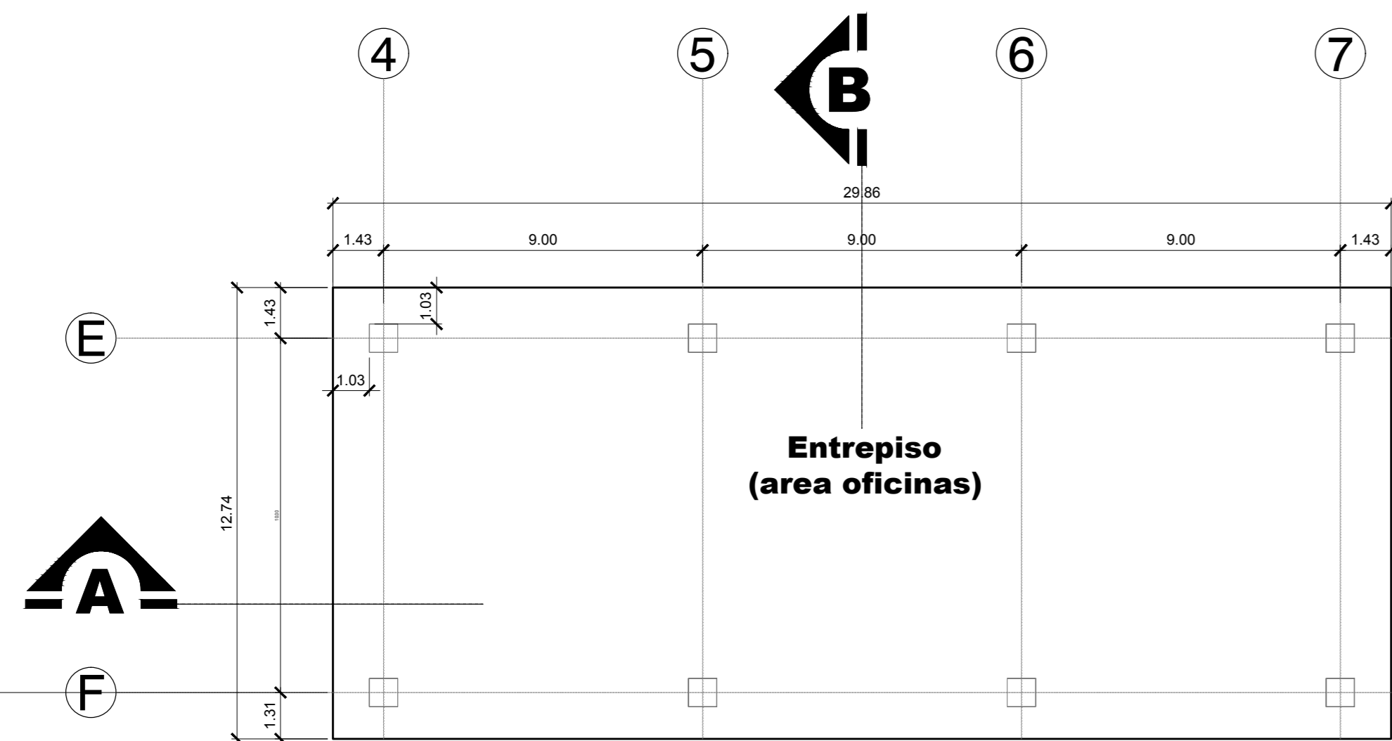
PLANTA DE DISTRIBUCIÓN NIVEL LOSA CONCRETO - NIVEL 0+36.63 ESC 1:150
