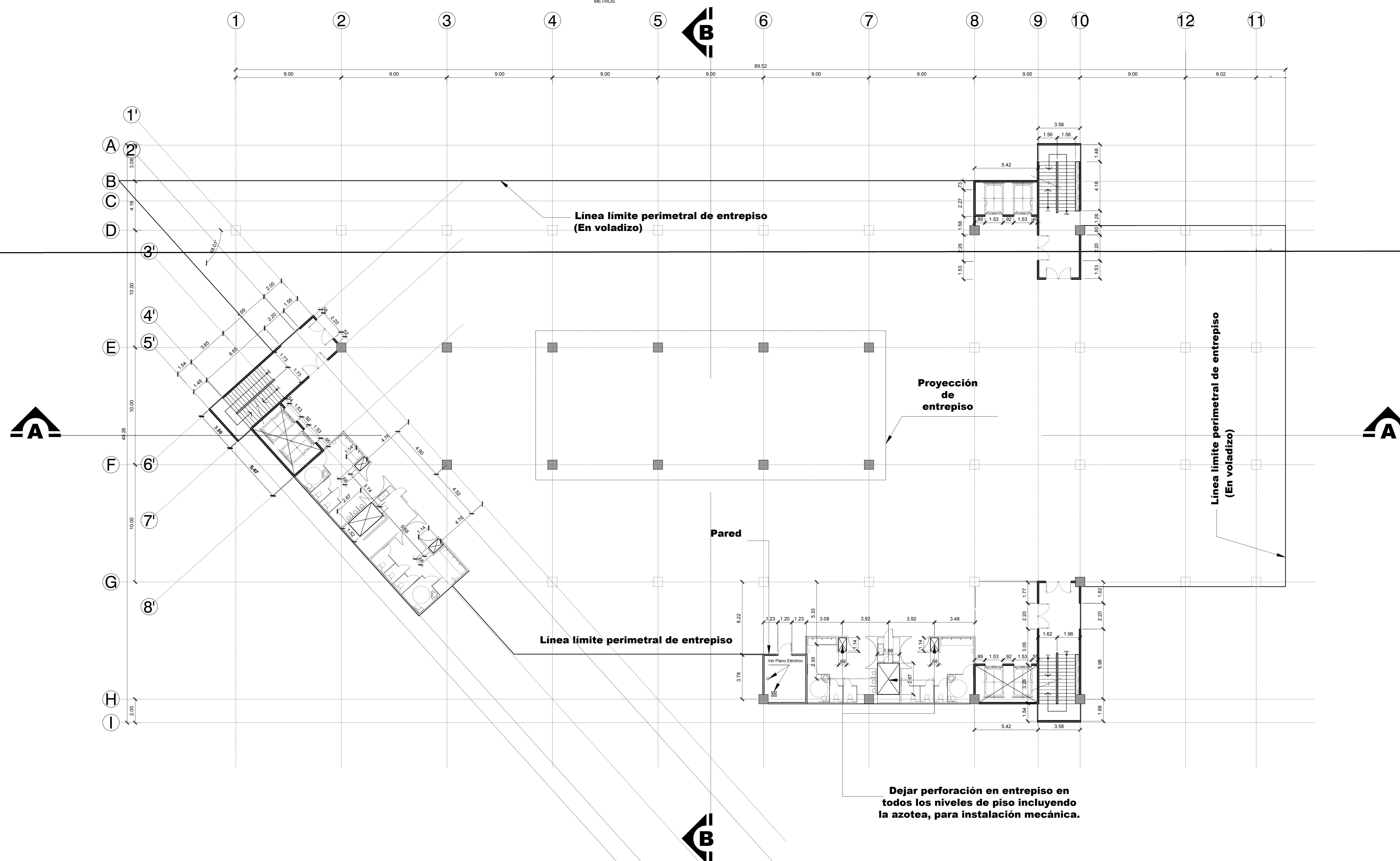
PLANTA DE DISTRIBUCIÓN NIVEL AZOTEA - NIVEL 0+32.56
