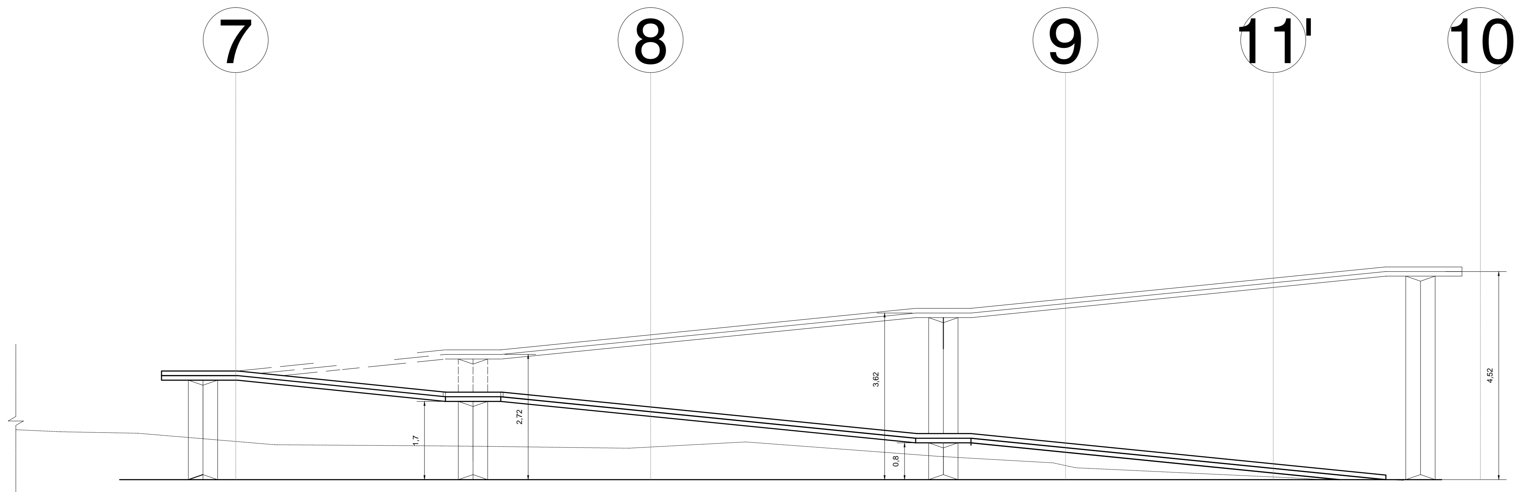
CORTE A-A ESC 1:50 METROS
