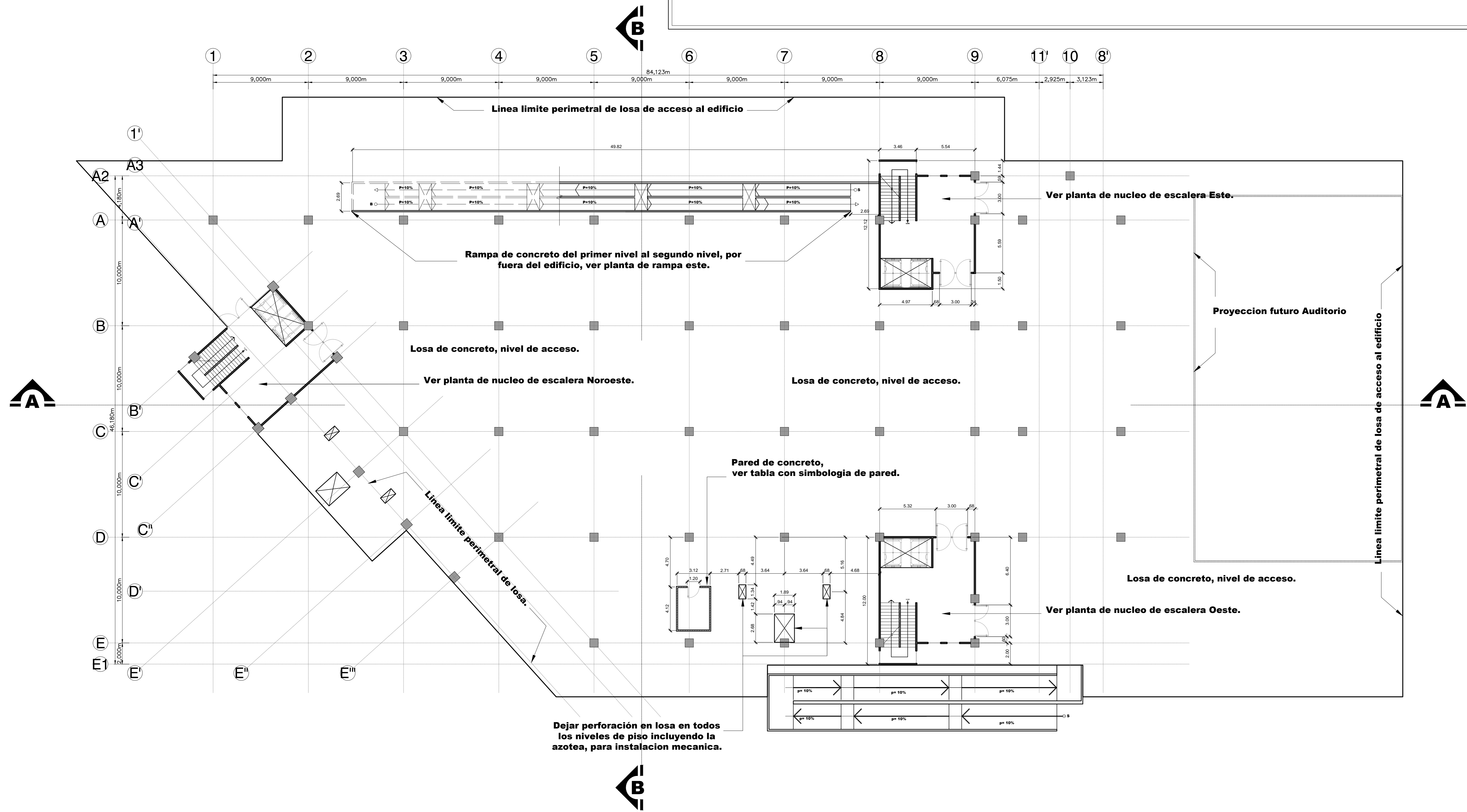
PLANTA DE DISTRIBUCIÓN PRIMER NIVEL - NIVEL 0+0.00 m
