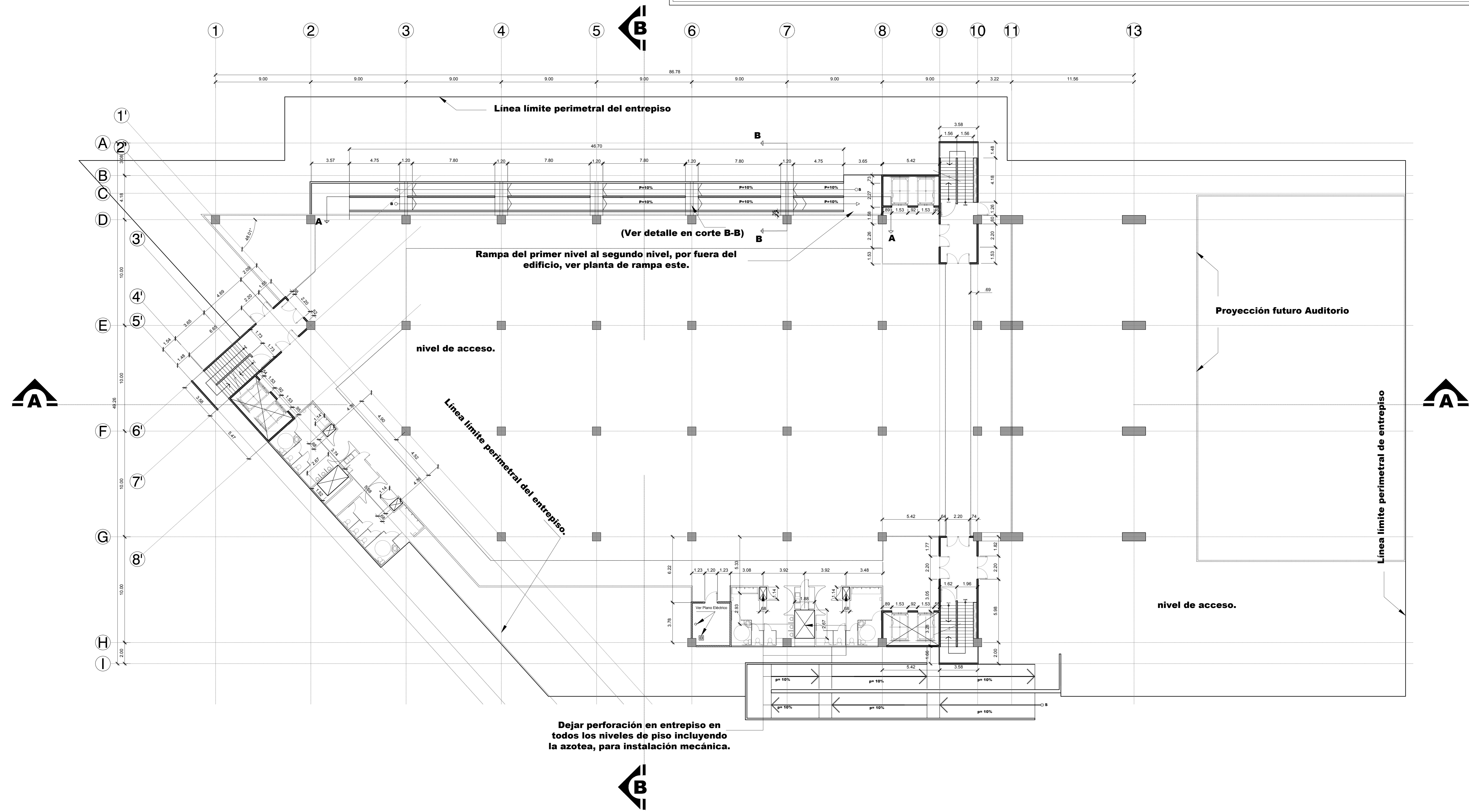
PLANTA DE DISTRIBUCIÓN PRIMER NIVEL - NIVEL 0+0.00 m ESC 1:150
