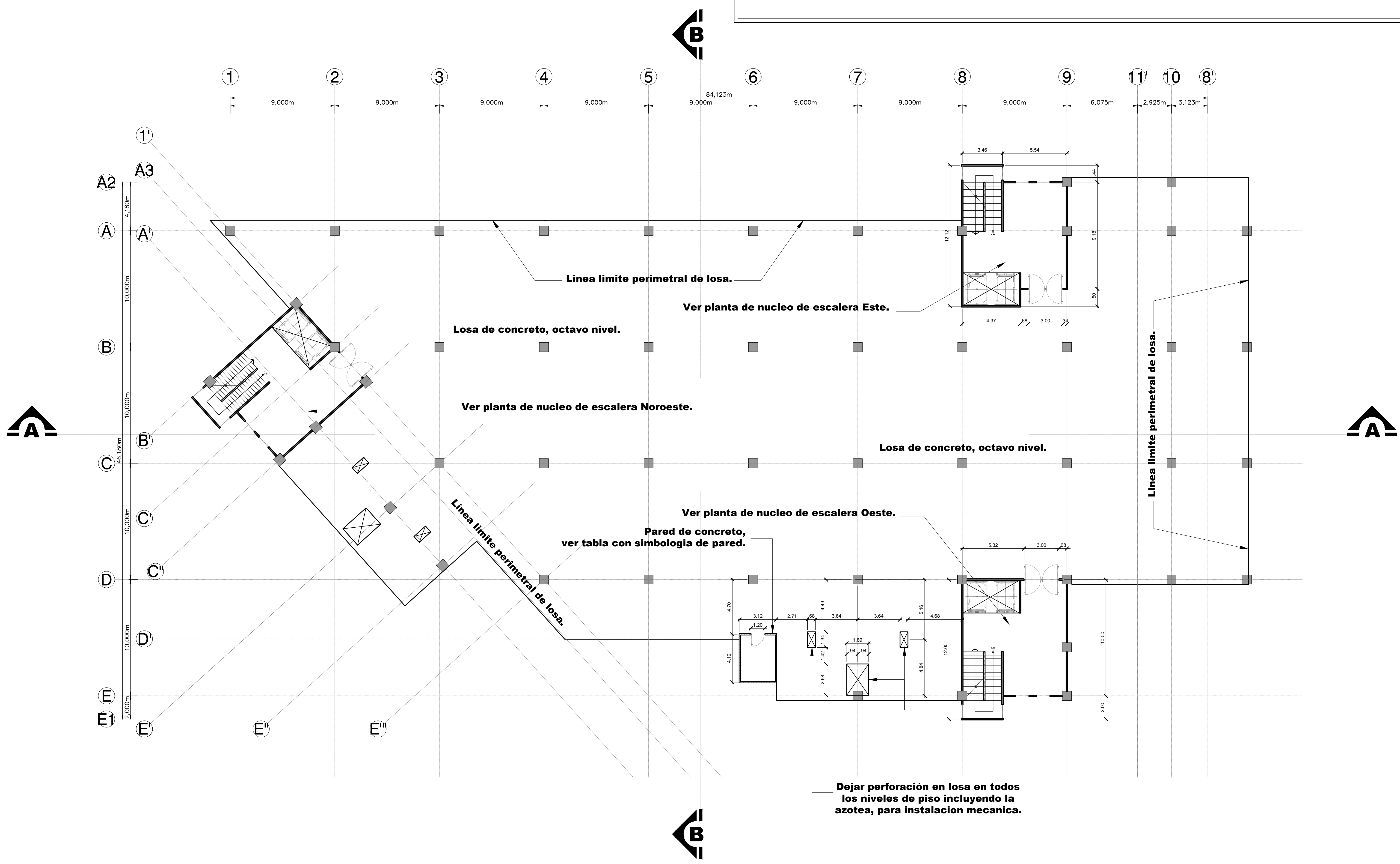
PLANTA DE DISTRIBUCIÓN OCTAVO NIVEL - NIVEL 0+28.49 ESC 1:150
