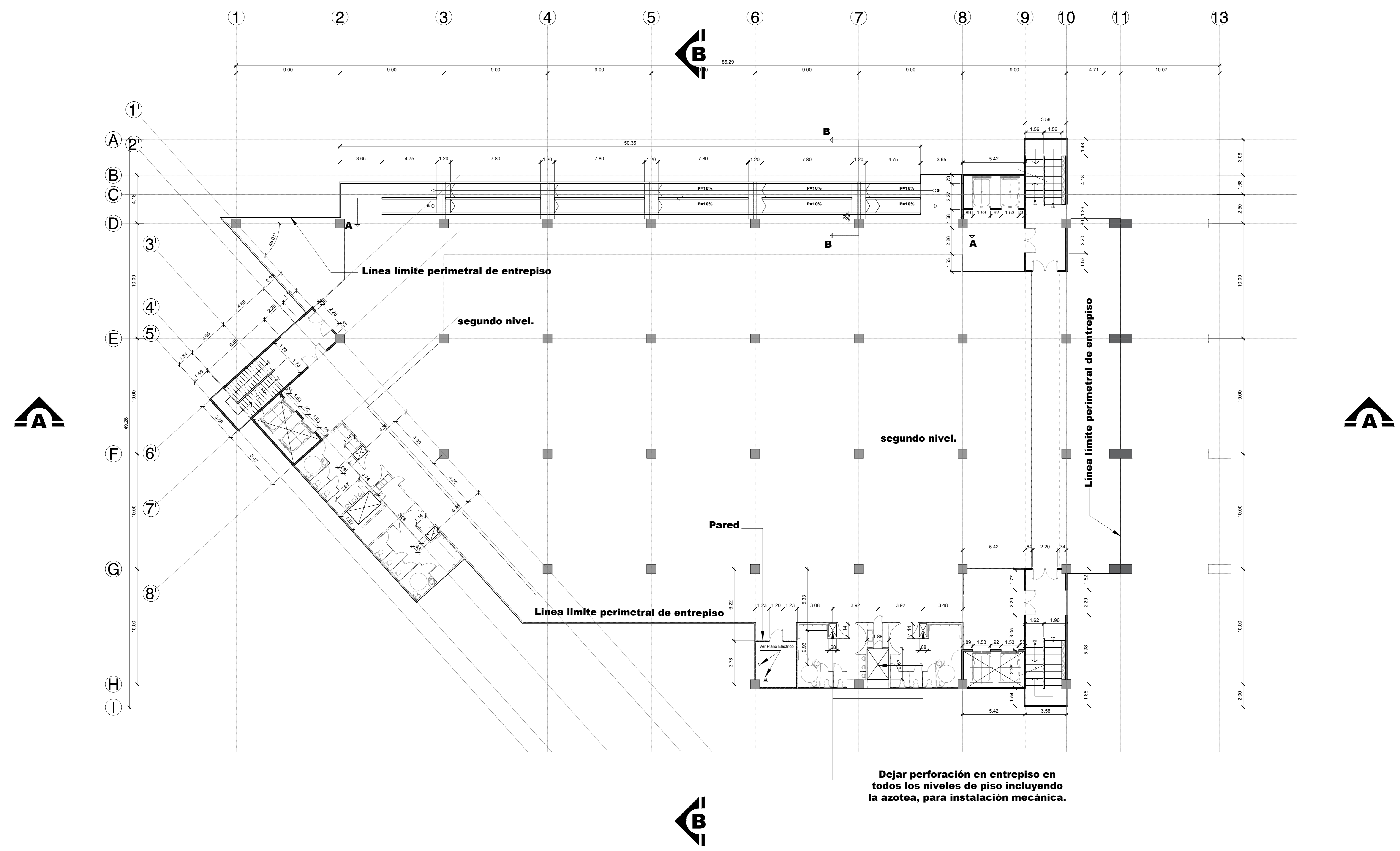
PLANTA DE DISTRIBUCIÓN SEGUNDO NIVEL - NIVEL 0+4.07 ESC 1:150
