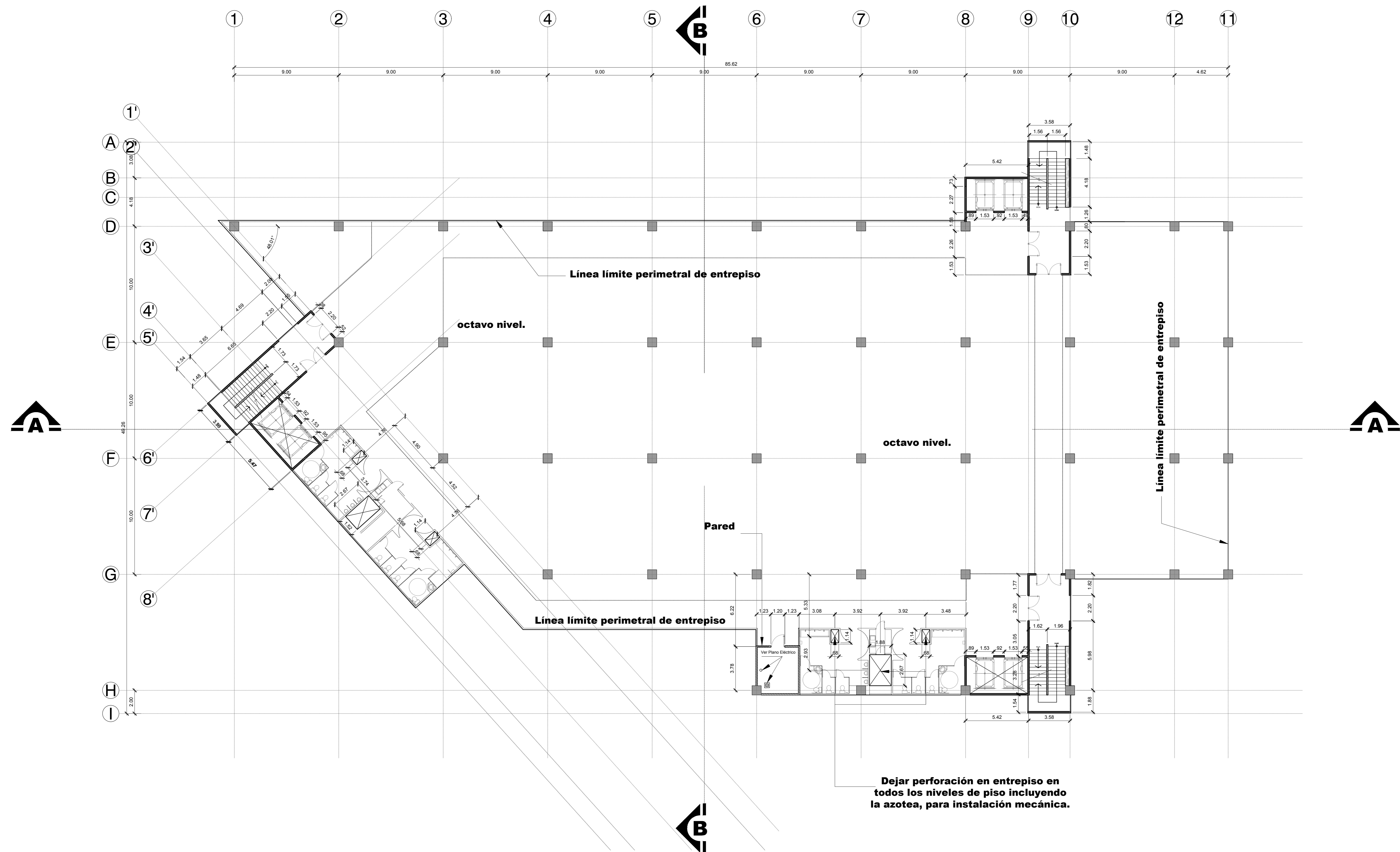
PLANTA DE DISTRIBUCIÓN OCTAVO NIVEL - NIVEL 0+28.49
