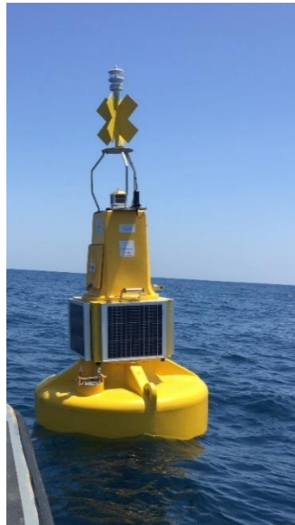
Figura 1 Boya SB138-P, diámetro de 1.75 m, altura focal de 2.9 m, color superficial amarillo con linterna de señal nocturna.
