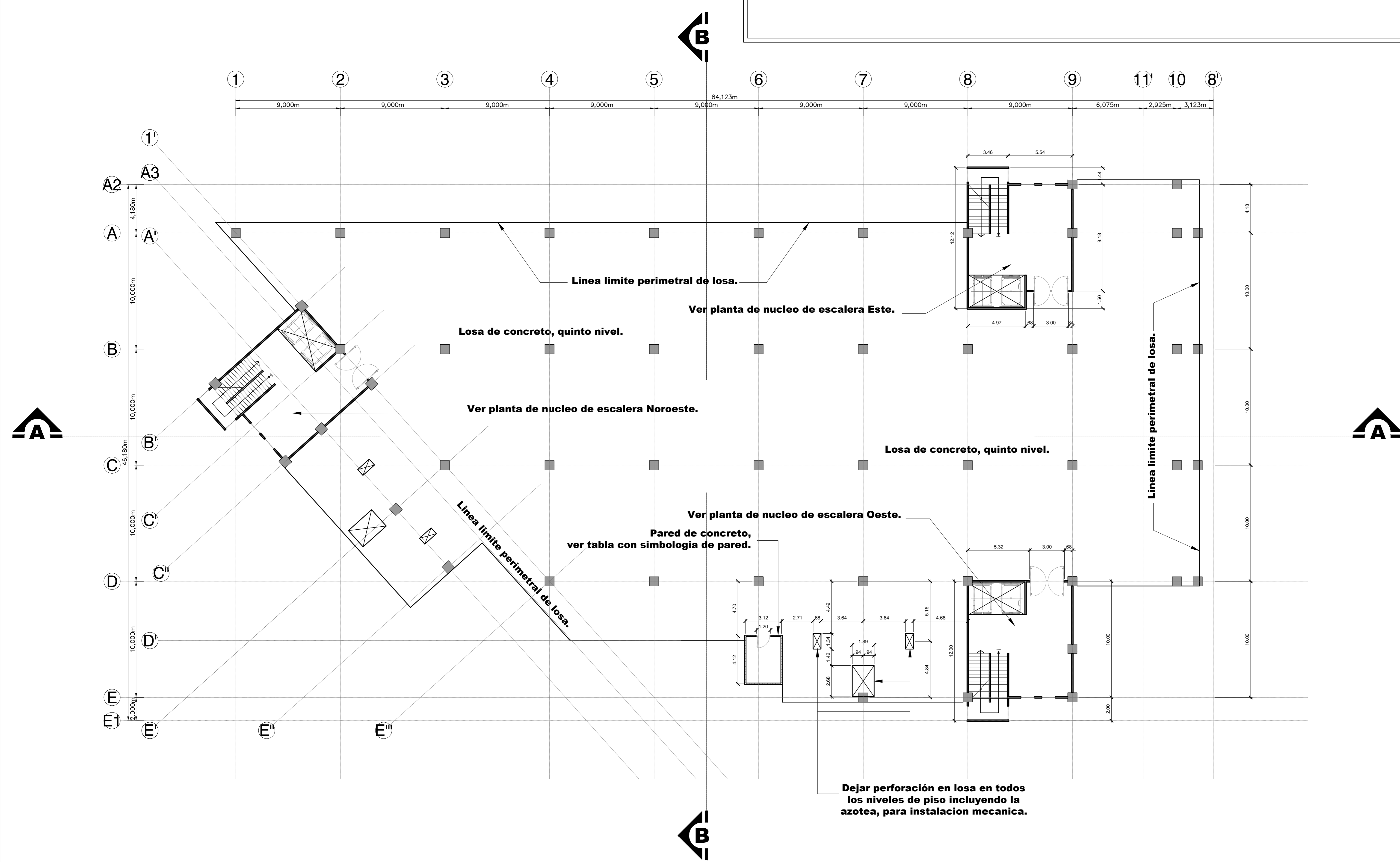
PLANTA DE DISTRIBUCIÓN QUINTO NIVEL - NIVEL 0+16.28
